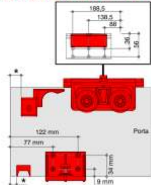
Sistemas de correr SS-150
