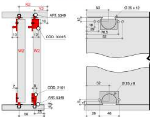
Sistemas de correr RO-80
