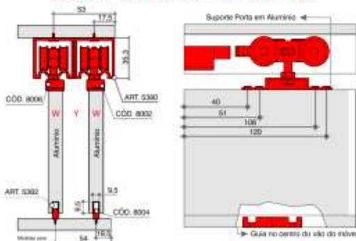
Sistemas de correr RO-80
