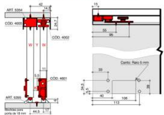
Sistemas de correr SS-150
